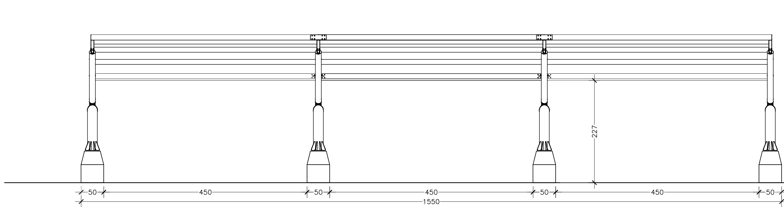
VISTA FRONTALE
