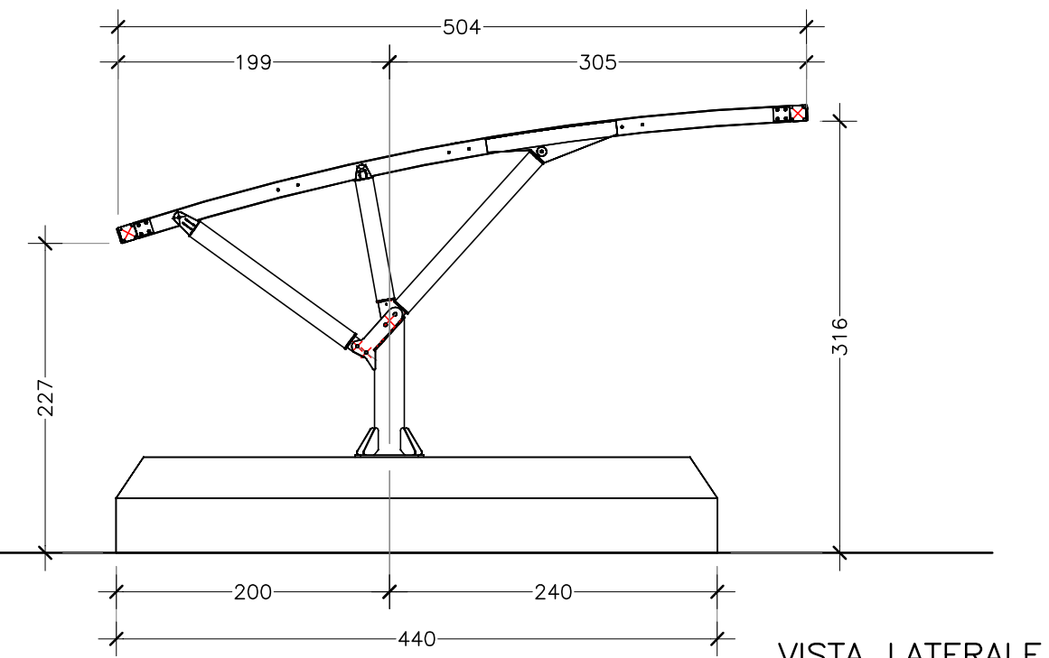
VISTA LATERALE
