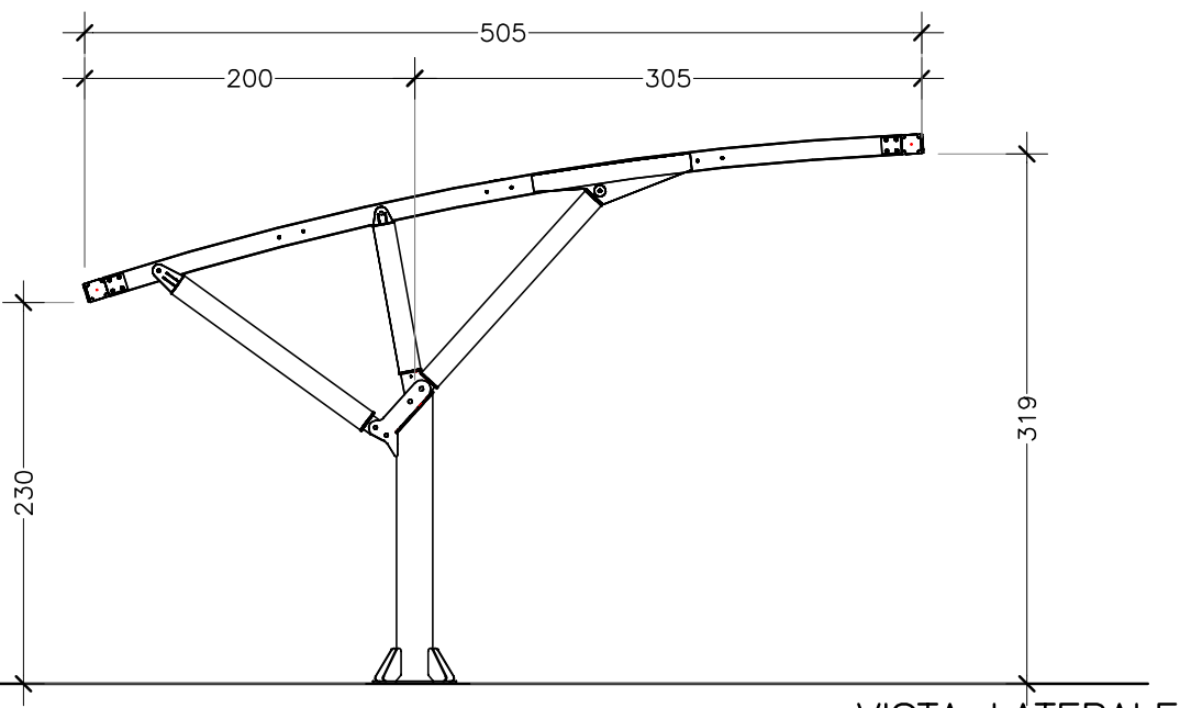
VISTA LATERALE
