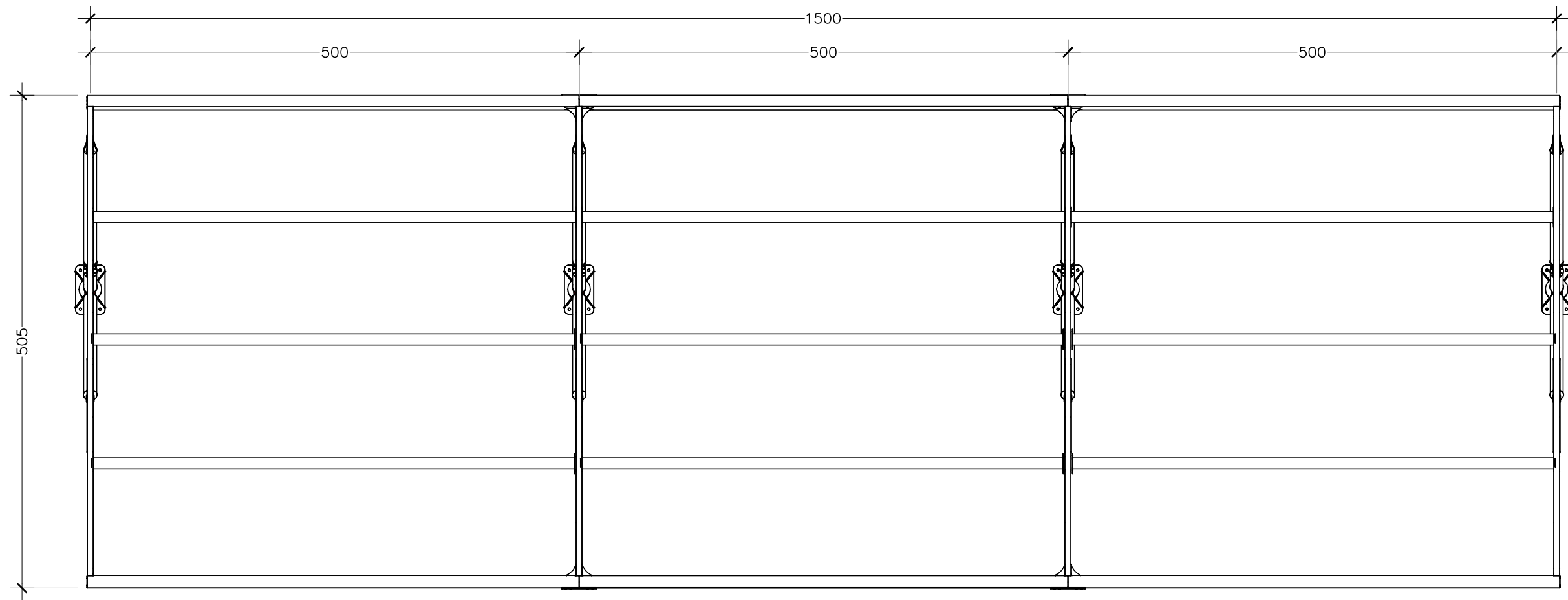
VISTA DALL'ALTO
